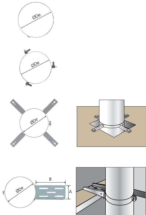
2 Para soporte mural interior (Ø350-Ø600) y exterior (Ø130-Ø600) For indoor (Ø350-Ø600) and outdoor wall clamps (Ø130-Ø600) Pour support mural intérieur (Ø350-Ø600) et extérieur (Ø130-Ø600)
