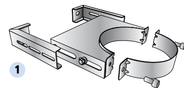
1 Para soporte mural interior y exterior (Ø130-Ø300) For indoor and outdoor wall clamps (Ø130-Ø300) Pour support mural intérieur et extérieur (Ø130-Ø300)
