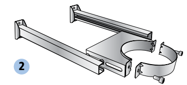
2 Para soporte mural interior (Ø350-Ø600) y exterior (Ø130-Ø600) For indoor (Ø350-Ø600) and outdoor wall clamps (Ø130-Ø600) Pour support mural intérieur (Ø350-Ø600) et extérieur (Ø130-Ø600)
