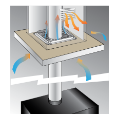
Distanciador fuego ventilado Ventilated firebreak Plaque écart au feu ventilée
